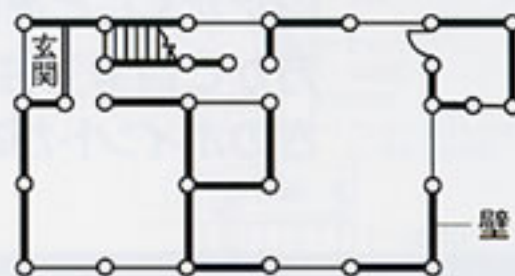
1階に壁が多い例
